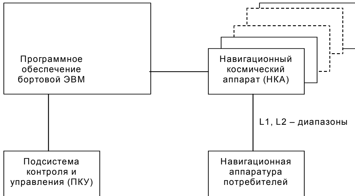
Рис. 3.1. Интерфейс НКА и НАП(АСН)
