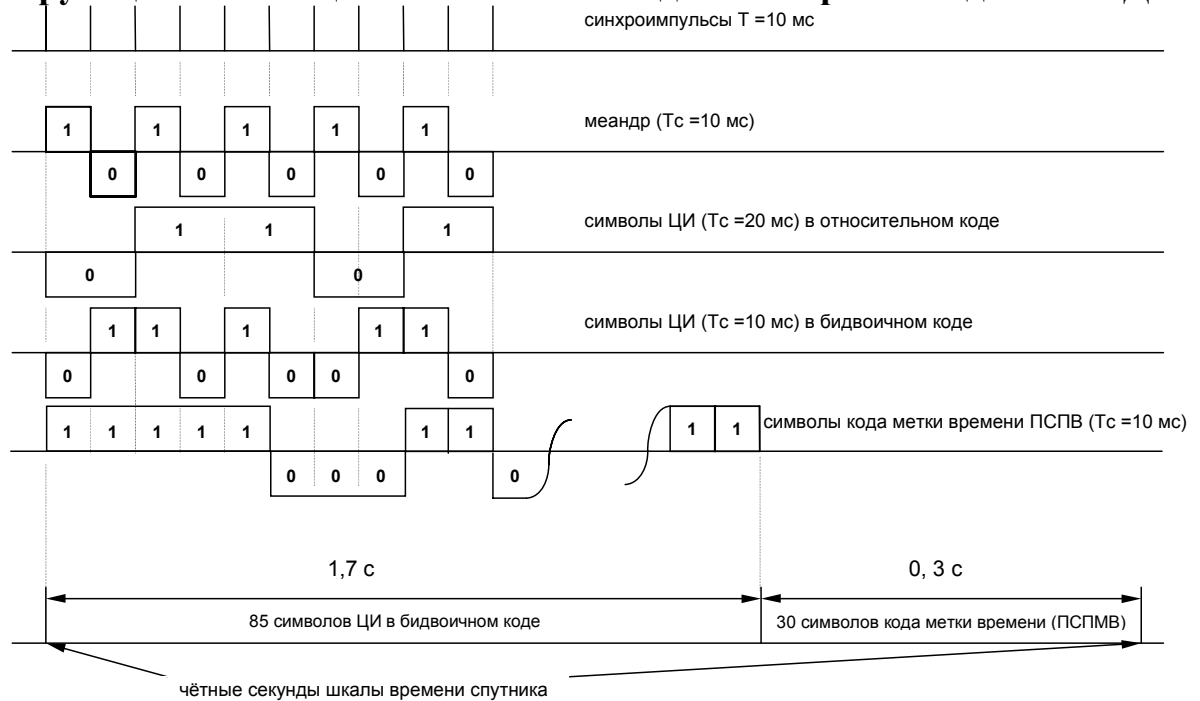
Рис. 3.5. Временные соотношения между синхроимпульсами модулирующего навигационного сигнала и дальномерным кодом ПСПД
